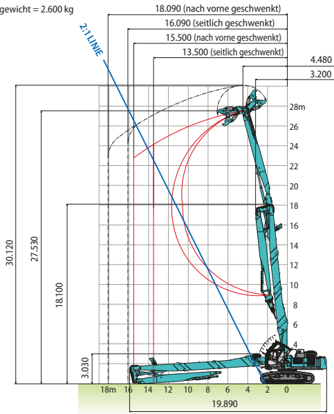
NEXT-Version mit ultra-langer NEXT-Arbeitsausrüstung: 8,7 m Stiel + 3,5 m Zwischenausleger
