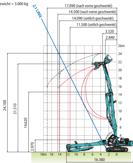
NEXT-Version mit ultra-langer NEXT-Arbeitsausrüstung: 6,1 m Stiel
