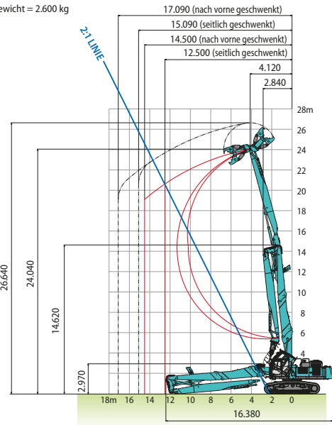
NEXT-Version mit ultra-langer NEXT-Arbeitsausrüstung: 8,7 m Stiel
