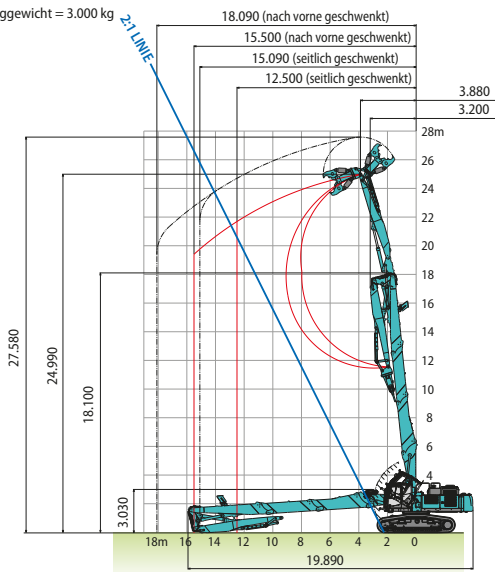
NEXT-Version mit ultra-langer NEXT-Arbeitsausrüstung: 6,1 m Stiel + 3,5 m Zwischenausleger
